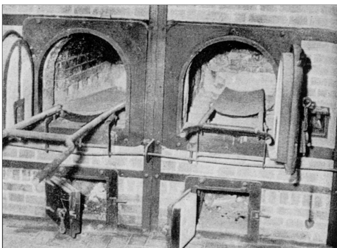
Abb. 1: Typischer Topf-Doppelmuffel-Einäscherungssofen in der Kriegsversion. Obere Schließknebel am Türrahmen fehlen. Vermutlich einzige veröffentlichte Innenaufnahme des Birkenauer Krematoriums, welches vier solcher Anlagen hatte. (VffG 2/98, S. 124)
