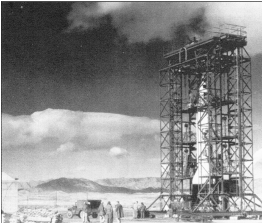
Aufnahme einer erbeuteten deutschen A-4/V-2 Rakete aus dem Jahr 1947. Im Rahmen des frühen US-Raketenprogramms wird dieses Beutestück gerade für den Start vorbereitet.
