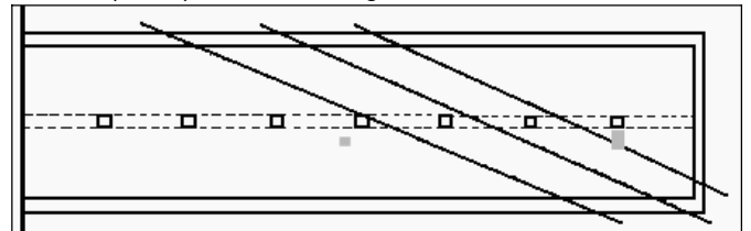
Abbildung 7: Querschnittszeichnung des Leichenkellers 1 von Krematorium II mit eingezeichneten Fluchtlinien als mögliche Aufenthaltsorte der drei Objekte aus Abbildung 5, sowie grau: ungefähre Lage und Größe der tatsächlich vorhandenen zwei Löcher.
