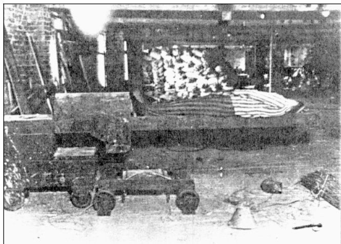
Abb. 14: Grifflose Montage- und Wartungslore mit Bombensplitter-Beschädigung. Aufgesetzte Montagehaube mit Profillehre. Darunter ausrangierter Eisenhunt zum Aschekasten-transport. Mann in Häftlingskleidung demonstriert auf dem Werksgelände der Maschinenbaufirma Topf die Lage von Ofenmauern bei der Muffelreparatur.
